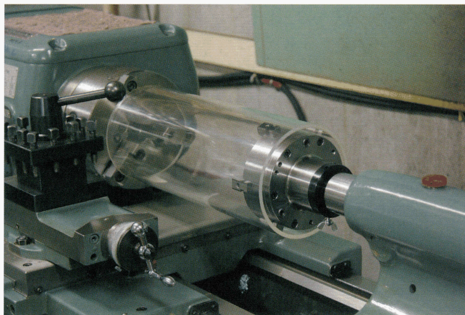
旋盤に取り付けたところ
