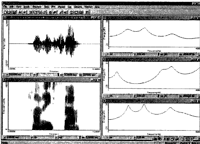
図 11 : h@risa の各母音に対する LPC (右列上段 : h@の@ ; 右列中段 : ri の i ; 右列下段 : sa の a)
