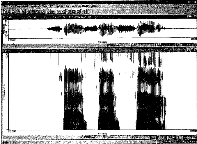
図 5-1 : sasasa (無意味語)
