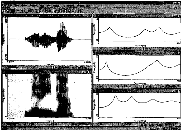
図 12：m@rida の各母音に対する LPC (右列上段：m@の@；右列中段：ri の i；右列下段：da の a)
