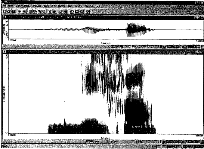
図 1-1 : b@dixa (冗談) ; (1a)@が無音で出現する例
