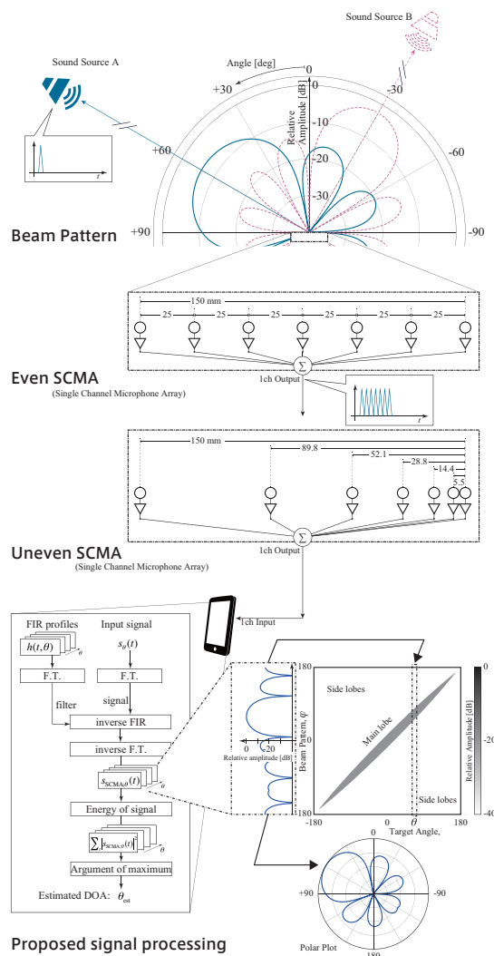
Fig. 1 単一チャンネルマイクロフォンアレー信号処理の概要
