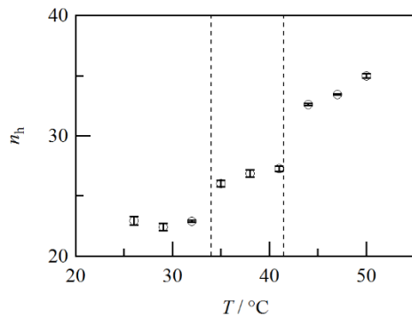
図 2 : DPPC の水和数の温度依存性 (低温からラメラゲル相—リップルゲル相—ラメラ液晶相。点線が転移温度を表す。)
