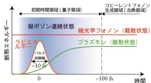
図1. 断熱エネルギー曲線の模式図
