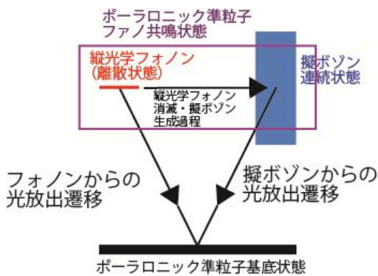
図 2. ポーロニック準粒子のファノ型相互作用の模式図
