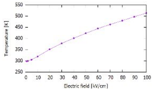
図 4. 自己無撞着に求めた温度の電場依存性
