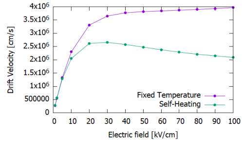
図 3. 熱の影響の有無によるドリフト速度の電場依存性
