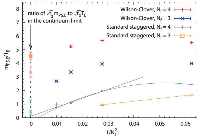
図 10: 臨界終点における \pi 中間子質量の格子間隔依存性。3、4 フレーバールンソン型フェルミオン作用の結果をそれぞれ青、赤色の点で示す。同様に、スタaggered型フェルミオン作用の結果をそれぞれ橙、紫色の点で示す。
