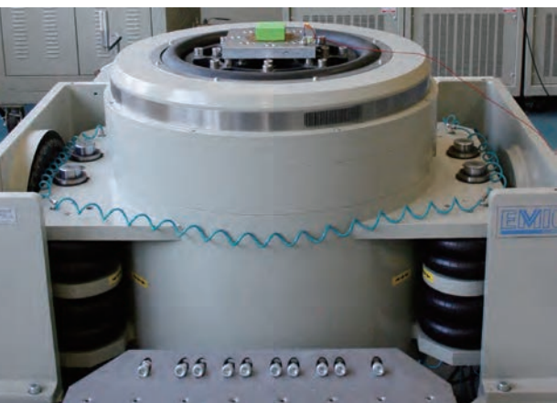
JAXA から譲り受けた振動実験装置(2月23日、筑波大学工学系H棟で) = 加藤優花撮影
