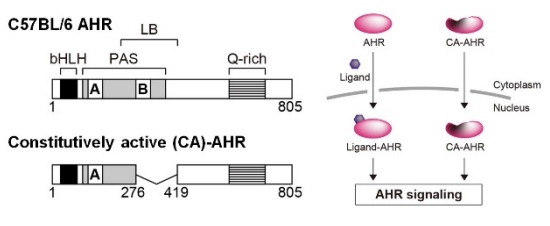
図 3. (左)C57BL/6 系統マウスの AhR と恒常活性型 AhR(CA-AhR)のタンパク質構造の模式図。(右)AhR は TCDD などのリガンドと結合することで核移行が可能となるが、CA-AhR はリガンドが無くても核へ移行し、下流シグナル伝達経路を誘導することができる。
