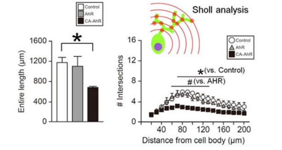
図 4. CA-AhR 発現による生後 14 日齢マウスの大脳錐体細胞における樹状突起の長さ (左) および複雑性 (右) の異常。
