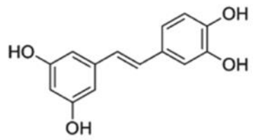
Piceatannol
