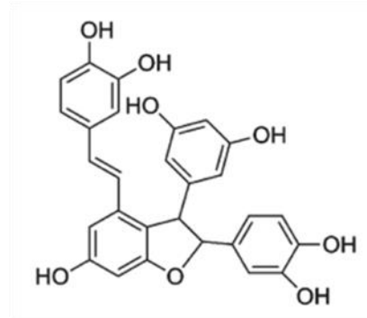
Scirpusin B
