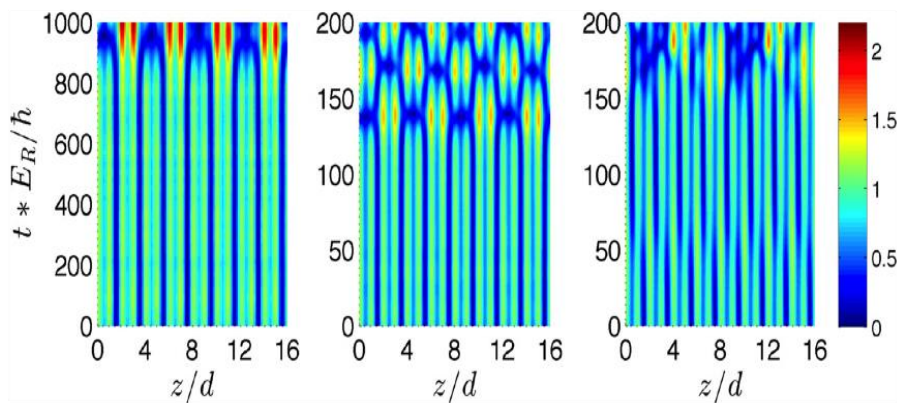
図2：TDBdG 計算による倍周期状態の安定性の検証。真ん中の図がユニタリ極限に対応し、左がBCS、右がBEC側に対応。
