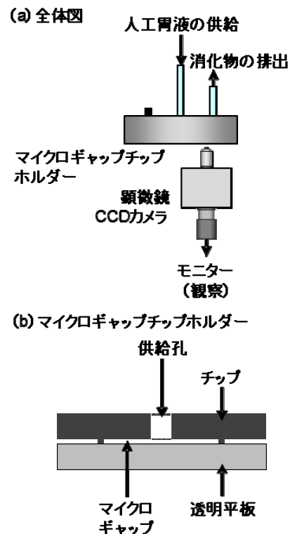
図 2 マイクロギャップ法による微小空間を利用した in vitro 胃消化評価システム
