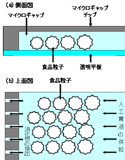
図 1 マイクロギャップ法の模式図
