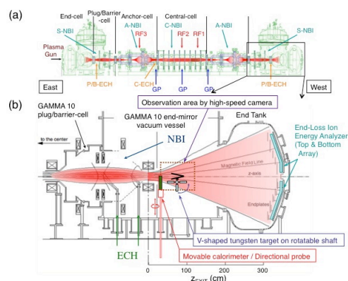
図 1 GAMMA 10 全体図 (a)、及び西エンド概略図 (b)
