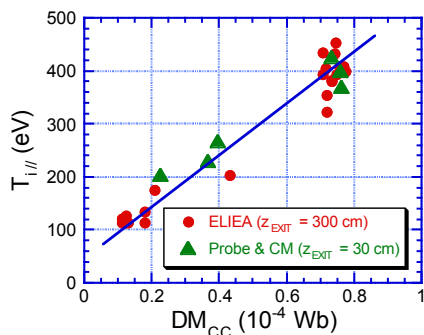
図 2 測定されたイオン温度とセントラル部プラズマの反磁性量の関係
