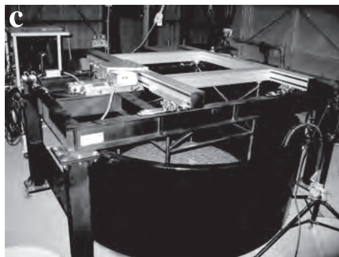
第1図 トラバース装置および円形水槽： (a) 側面図，(b) 上面図，(c) 写真.
