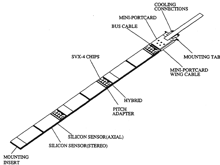
図 6: SVX IIb 用ステイブの模式図。ステイブは、片面シリコンセンサーを両側から張り合わせた構造になっており、12 枚のセンサーから構成されている。
