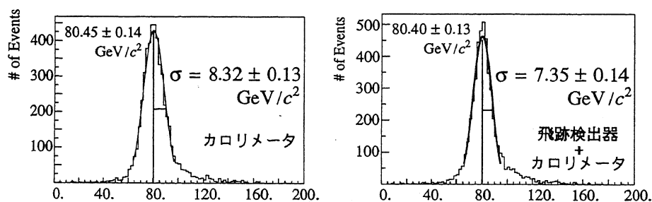
図 8: カロリメータの情報のみを用いた場合 (左) と飛跡検出器とカロリメータの両方の情報を用いた場合 (右) の W ボゾンの質量分布
