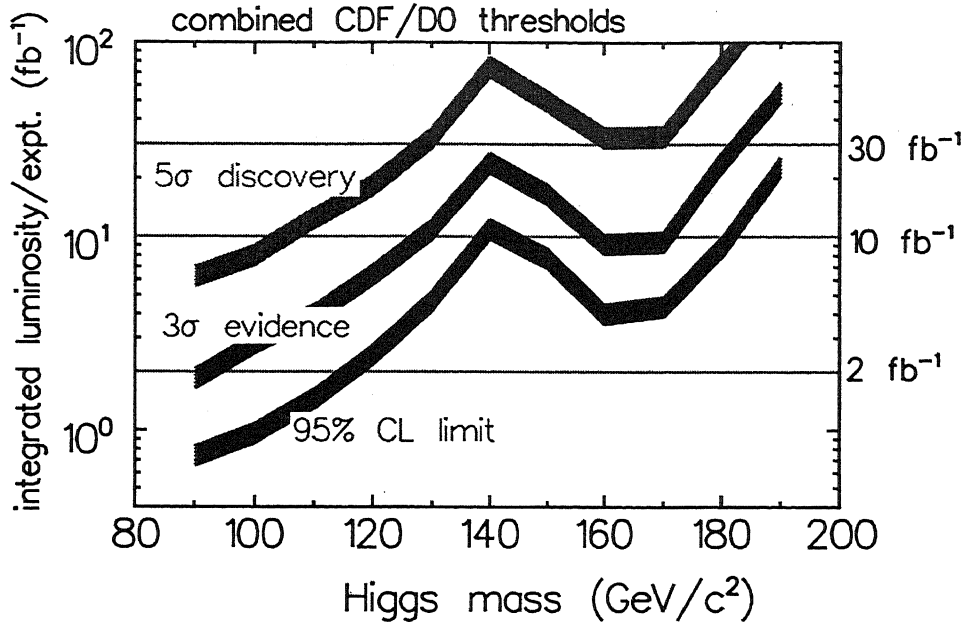
図 5: テバトロンでの標準模型ヒッグス粒子探索に必要なデータ量 (積算ルミノシティー) をヒッグス粒子の質量の関数として示したもの. 3本の帯は上からそれぞれ, (a) 5標準偏差の統計的有意さをもって発見する, (b) 3標準偏差の有意さで存在の証拠を示す, (c) もし存在しない場合に95%の確度で排除する, ために必要なデータ量に対応する.
