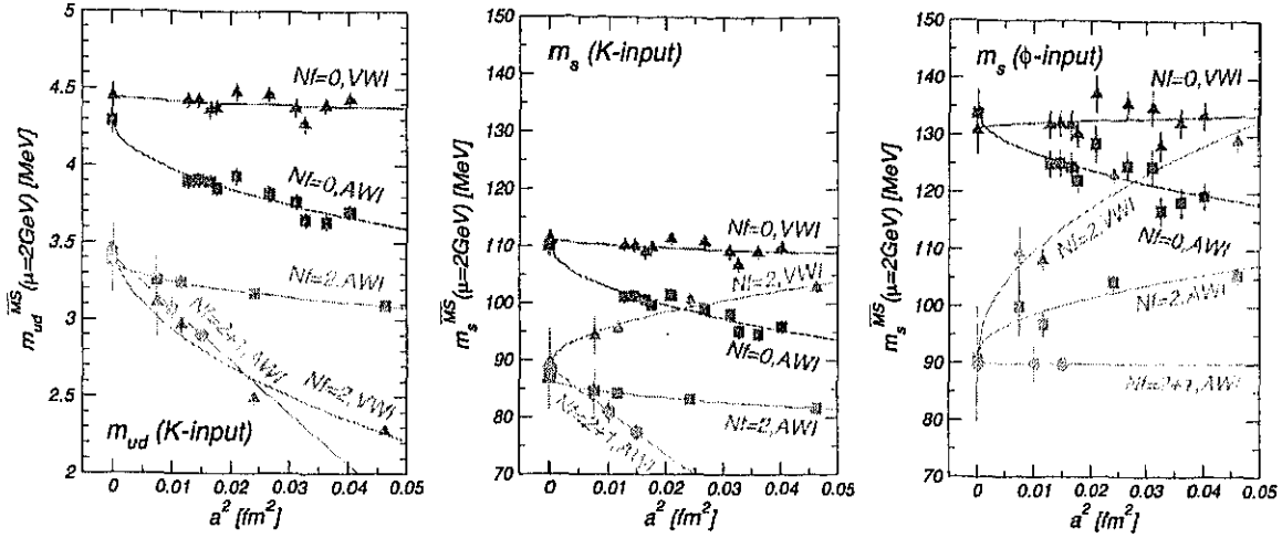
図 2: 軽いクォークの質量の連続極限への外挿。左が up と down クォーク (K-input)、中央が strange クォーク (K-input)、右が strange クォーク ( \phi -input)。くり込みスキームは \overline{MS} ( \mu = 2 \text{ GeV} )。青○が N_f = 2 + 1 の値。比較のため N_f = 2 (黄) とクエンチ近似 (茶) の値も図示した。AWI, VWI はクォーク質量の定義の違いで、両者は連続極限で一致すべきものである。 N_f = 2 + 1 では AWI 定義だけを図示している。現段階では連続極限で N_f = 2 + 1 と N_f = 2 の結果は同程度となっている。
