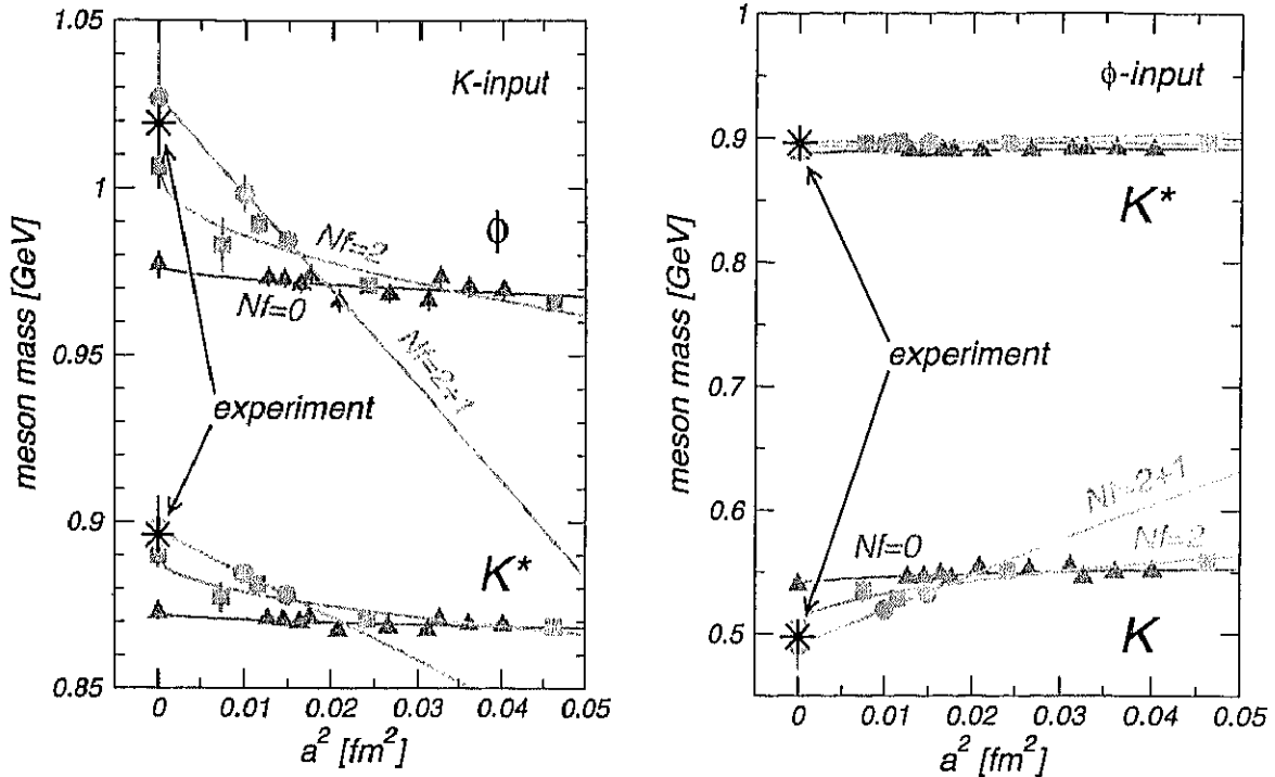
図 1: 軽い中間子質量スペクトルの連続極限への外挿。青○が N_f = 2+1 の値。比較のため N_f = 2 (黄□) とクエンチ近似 (茶△) の値も図示した。K-input、 \phi -input は物理点を決定するときの入力としてそれぞれ K 中間子、 \phi 中間子を使ったことを意味する。 N_f = 2+1 の中間子質量スペクトルは連続極限で実験値を再現する。
