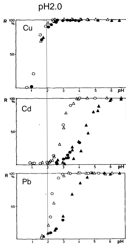
図 3-5-2 pH における金属(Cu、Cd、Pb)の吸着効率 [10]
