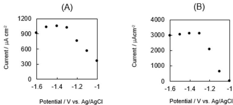
図 2-17-1 堆積電位と ASV の酸化電流の関係 (A) 1000 ppb Cd 2+ (酢酸 pH 5.0)、(B) 1000 ppb Pb 2+ (クエン酸 pH 2.0)
