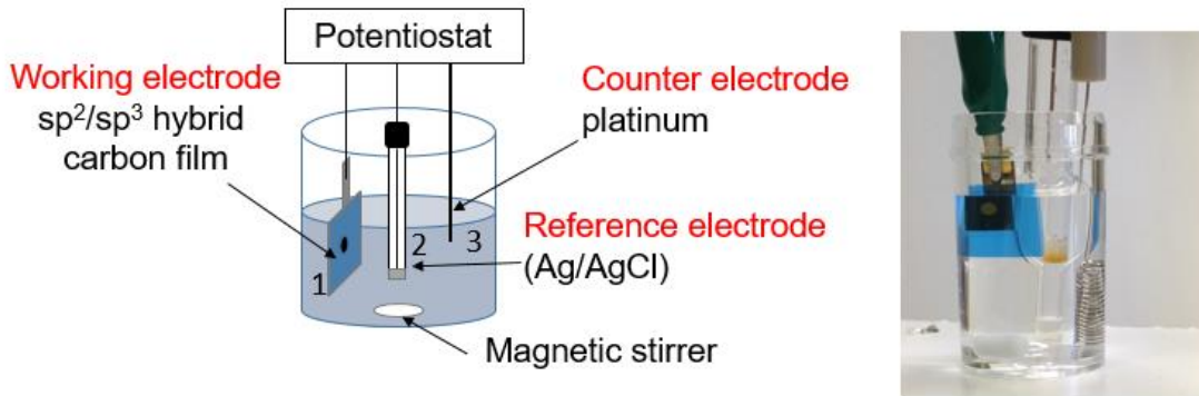
図 2-10-1 ASV 測定 of 電気化学的測定セル
