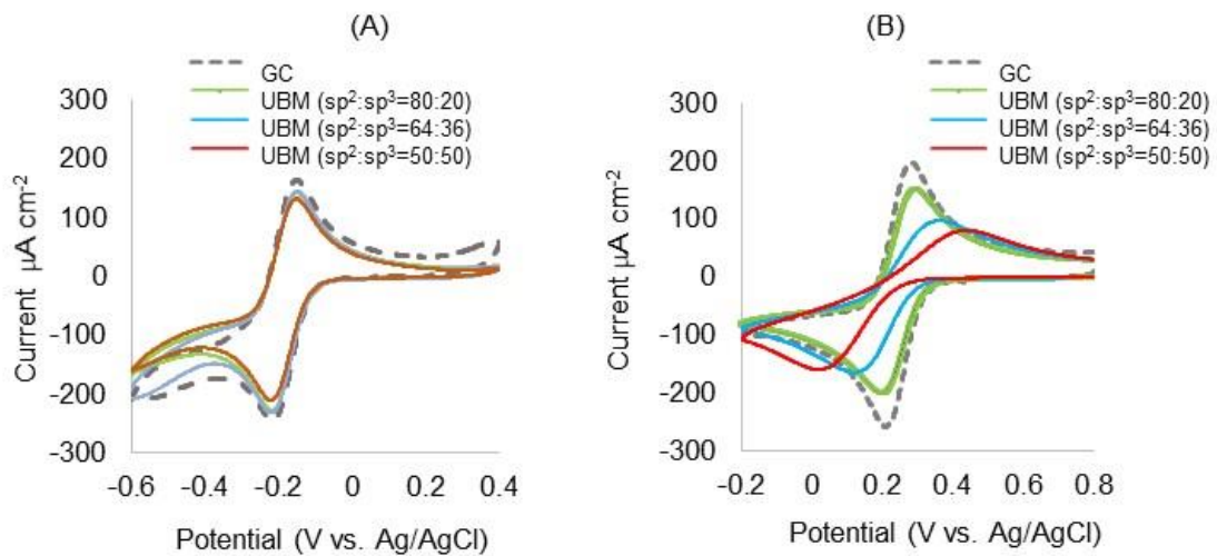
図 2-12 サイクリックボルタモグラム
