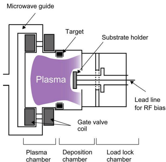
図 2-4 ECR スパッタ装置の概略図 [16]
