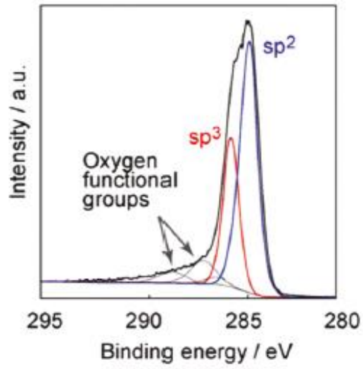
図 2-5 ECR ナノカーボン薄膜の XPS データ [17]
