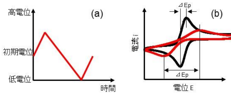
図 2-11 CV 測定 of 電位スweep の例(a)と CV 応答の例(b)
