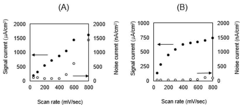
図 2-17-2 UBM (50:50)を用いたスキャン速度に対するシグナルとノイズ電流の関係 (A) 100 ppb Cd (酢酸 pH 5.0)、(B) 100 ppb Pb (クエン酸 pH 2.0)、●:シグナル電流、○:ノイズ電流
