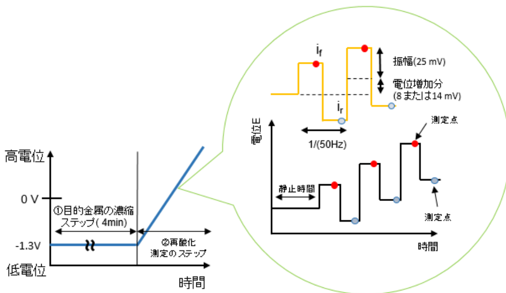
図 2-10-2 ASV 測定 of 条件
