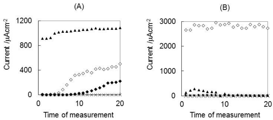
図 2-14 様々な測定溶液における 1000 ppb の電流値と繰り返し性、Cd 2+ 、(B) Pb 2+ 、×EDTA (pH 5.0)、 ◆クエン酸緩衝溶液(pH 5.0)、◇クエン酸緩衝溶液(pH 2.0)、▲ 酢酸緩衝溶液(pH 5.0)
