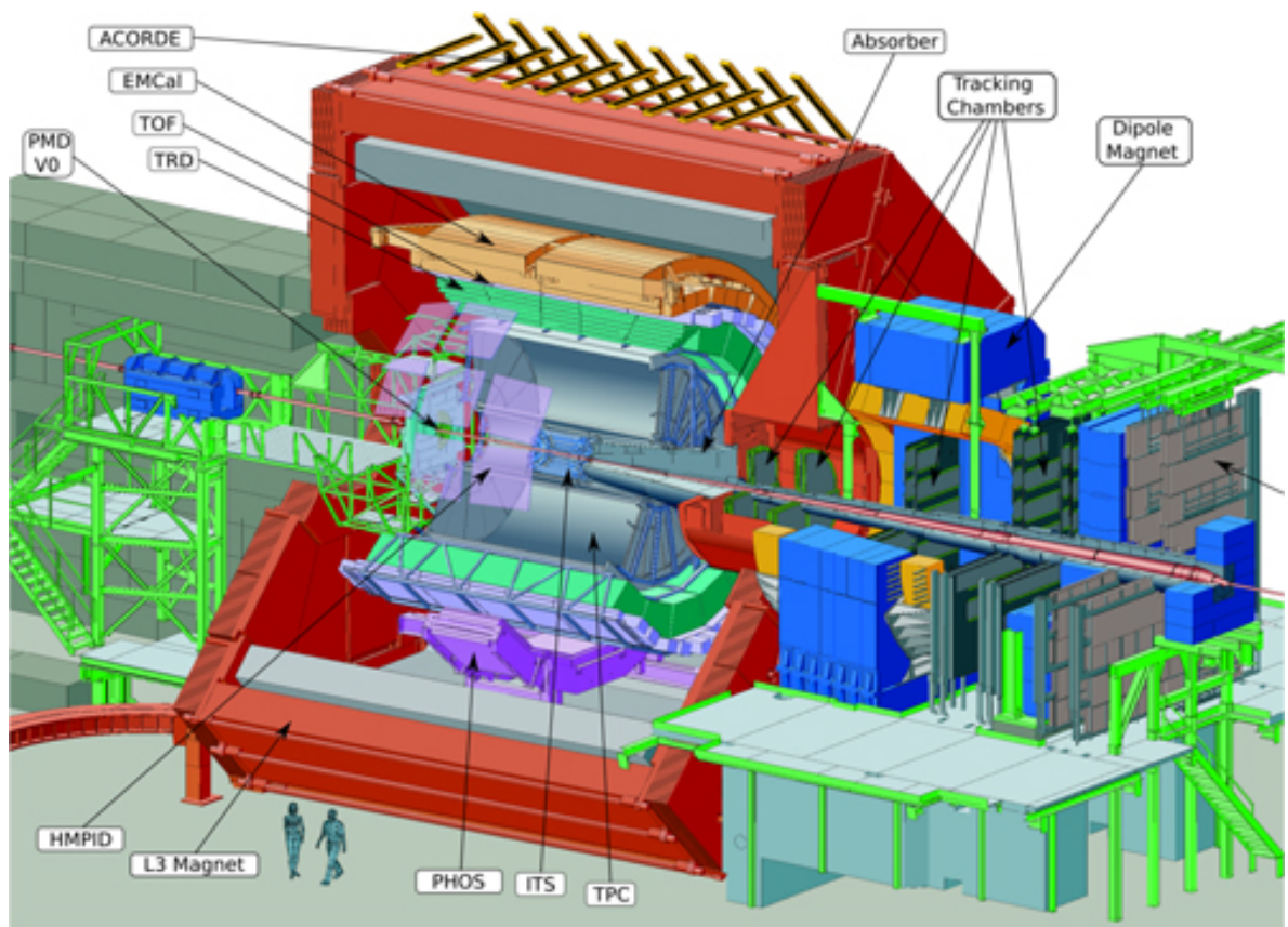
Fig. 2.2.1: ALICE detector
