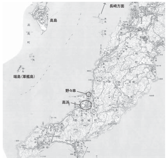
図1 調査地位置
