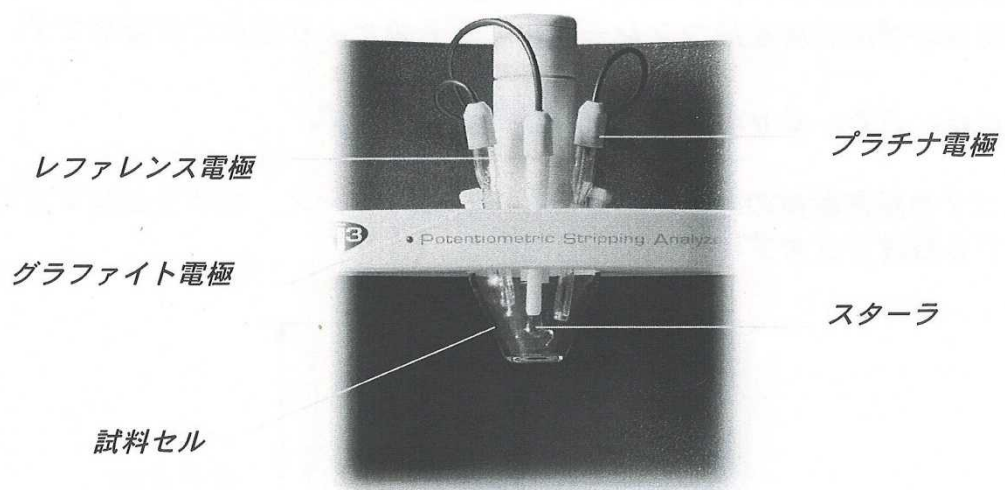
図 2. ION 3 の電極
