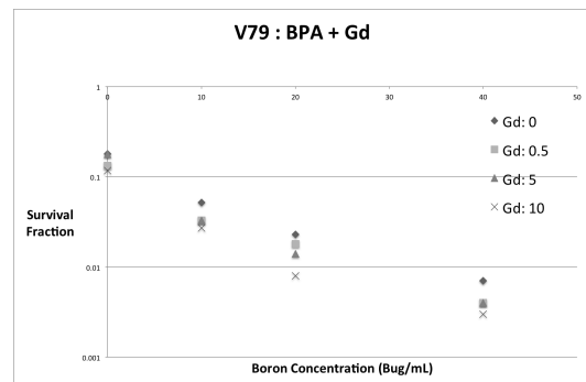
Figure 1. ホウ素ガドリニウム併用中性子捕捉反応 C6 (上段), V79 (下段)
