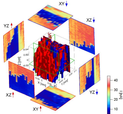
図 5. Si-DEB 単一分子接合の 3D 伝導計測結果
