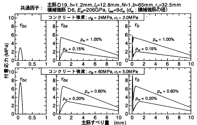
図10 局所付着応力-すべり量関係
