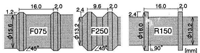
図 1 切削加工した鉄筋の節形状
