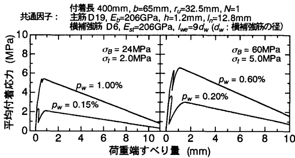
図 11 平均付着応力-荷重端すべり量関係
