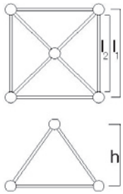
図 11 試験体形状
