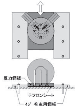
図 13 支点部詳細
