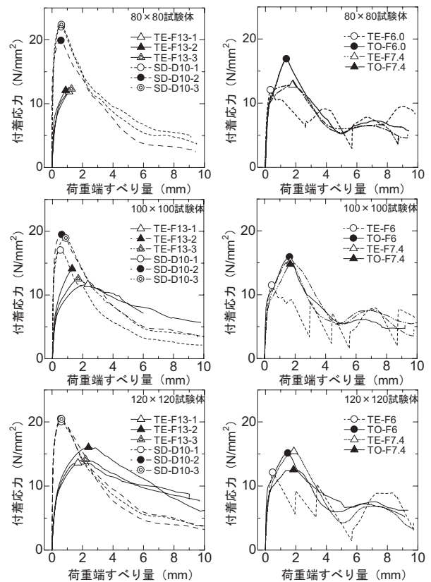
図5 付着応力-すべり量関係
