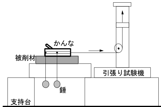
図 3. 実験装置
