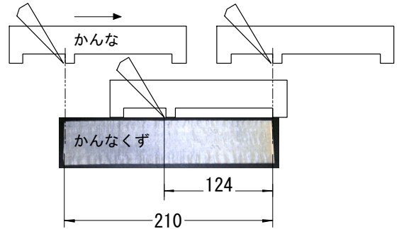
図 6. かなな下端位置とかななくずとの関係 (mm)
