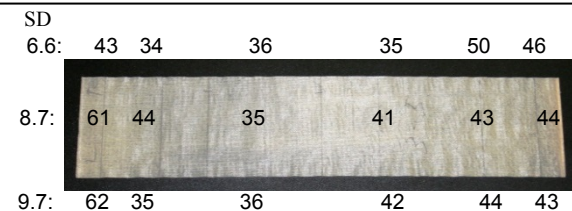
3点接触 [4×6=24kgf] 時の切りくず(μm)【図8-く】
