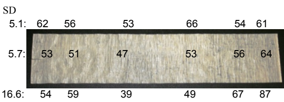
2点接触 [3×6=18kgf] 時の切りくず(μm)【図8-し】
