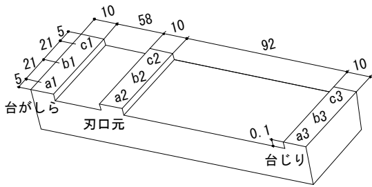
図 2. かなな下端面測定位置 (mm)
