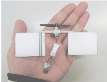
図6：シングルロータ飛行ロボット Switchou
