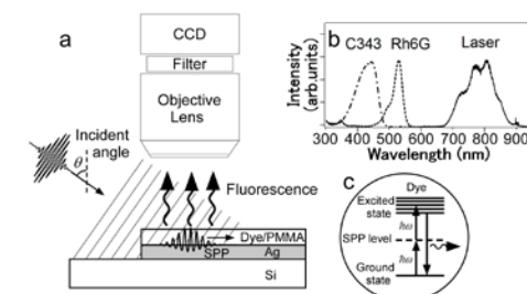
Fig.1 二光子蛍光顕微鏡法による表面プラズモン波束イメージングの実験法概略。
