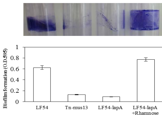
Fig. 5 各種 lapA 変異株によるバイオフィーム形成
