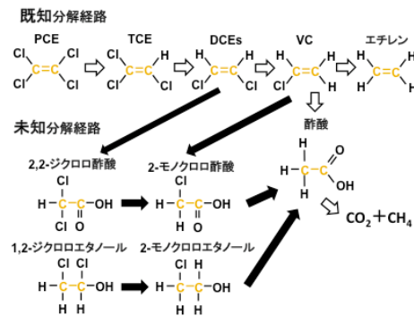
Fig. 3 テトラクロロエチレン分解経路
