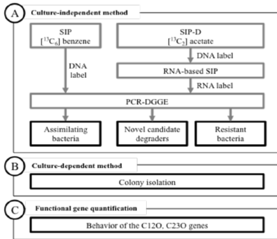
Fig. 2 ベンゼン分解菌ネットワークの解析法
