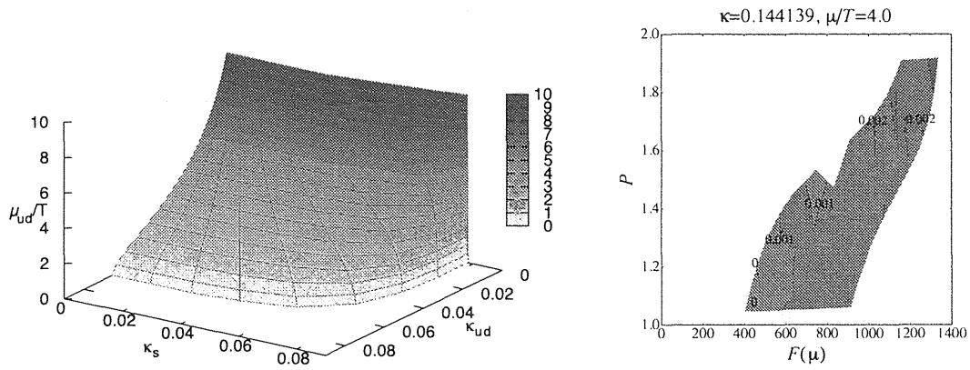
図 10: ヒストグラム法による QCD の有限温度相構造の研究。(左) 重クォーク領域における N_f = 2+1 QCD の臨界面 (論文 25)。 u, d クォークにだけ化学ポテンシャル \mu_{ud} がかかり、 s クォークにはかかっていない場合の結果。ホッピングパラメータ \kappa はクォーク質量の逆数にはほぼ比例する量で、 \kappa_s = 0 は m_s = \infty 、 \kappa_{ud} = 0 は m_u = m_d = \infty に対応する。図の臨界面の向こう側は有限温度 QCD 転移が 1 次相転移で、手前はクロスオーバーになっている。(右) クォークが軽い N_f = 2 QCD の相構造の研究 (論文 26)。有効ポテンシャルの 2 階微分を、物理量 P (ブラケット) と F (クォークの自由エネルギーに関する量) の関数として示す (プレリナリ)。この量がゼロになる点で、クロスオーバーが 1 次相転移になる。
