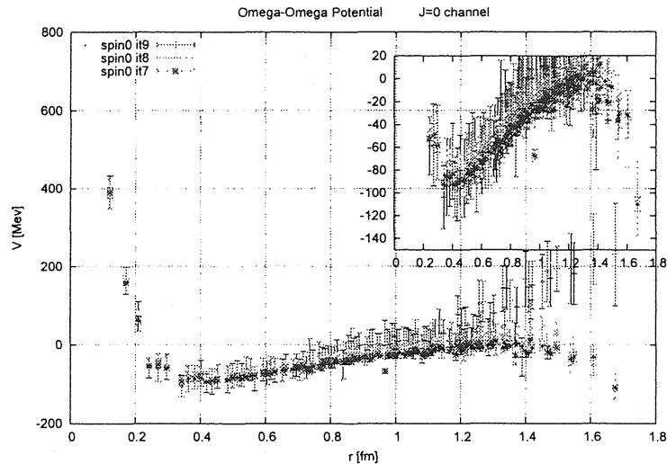
図 7: J = 0 である \Omega - \Omega 間のポテンシャル V[\text{MeV}] 。横軸はバリオン間の距離 r[\text{fm}] 。
