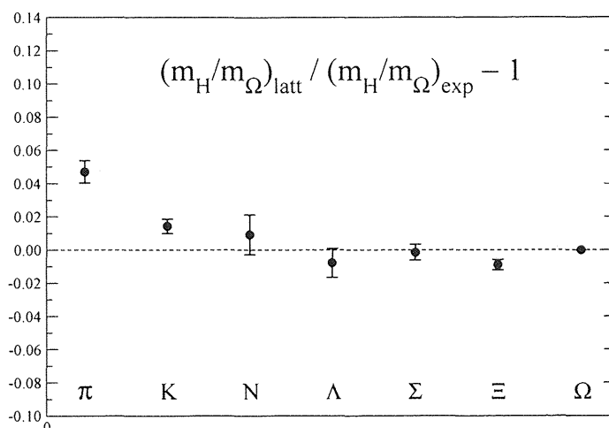
図 2: ハドロン質量と実験値との比較。
