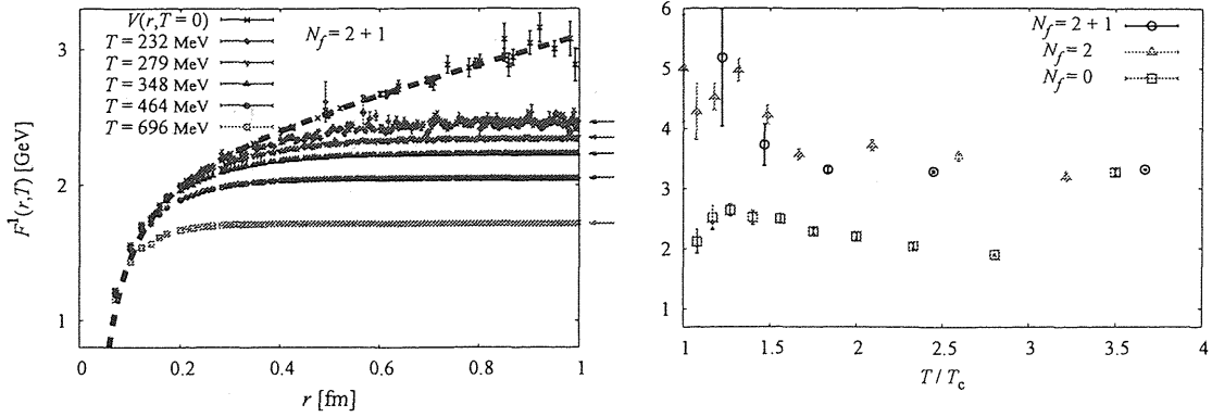
図 9: 固定格子間隔アプローチによる静的クォークの自由エネルギーの研究 (論文 22)。(左図) N_f = 2+1 QCD における Q\bar{Q} カラー 1 重項チャンネルの静的クォーク自由エネルギー。ゼロ温度 ( T = 0 ) の自由エネルギーはウイルソン・ループの測定により、有限温度の自由エネルギーは 2 個のポリアコフ・ループの相関から評価した。固定格子間隔アプローチでは、定数くりこみの調整無しに、自由エネルギーが短距離で温度に依らないことを直接示すことが出来る。右端の矢印は、ポリアコフ・ループ 1 個の期待値から期待される自由エネルギーの遠距離極限の漸近値。(右図) デバイ遮蔽質量 m_D(T) のフレーバー数依存性。縦軸は m_D(T)/T 、横軸は T/T_c 。 T_c は相転移温度で、 N_f = 2+1 では 190MeV を仮定した。
