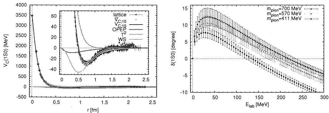
図 4: (左) 2+1 flavor 格子 QCD で計算された核力 (spin-singlet 中心力) のフィットの結果 ( m_\pi \simeq 570 MeV) (右) これを使った ^1S_0 の散乱位相差 ( m_\pi \simeq 411, 570, 700 MeV)。
