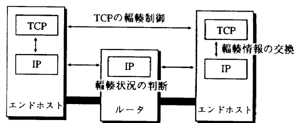
図1 明示的輻輳通知
