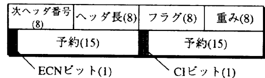
図 3 提案する拡張輻輳通知ヘッダ
