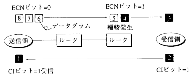
図 2 RED ゲートウェイ方式の輻輳通知
