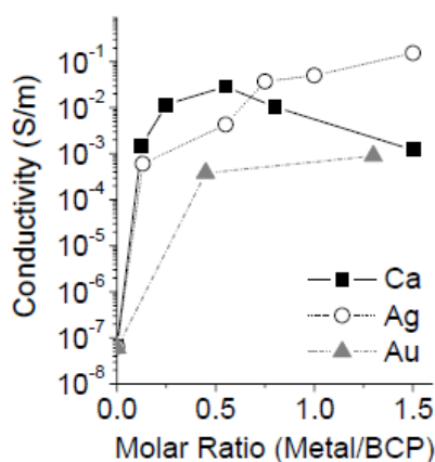
図 2. 金属添加 BCP 膜の電気伝導度
