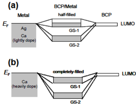
図4.金属添加BCP膜のエネルギー状態図
