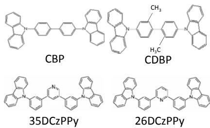
図5.カルバゾール系分子
