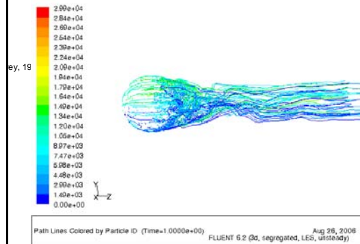
図 4 サッカーボール回りのパスライン。
