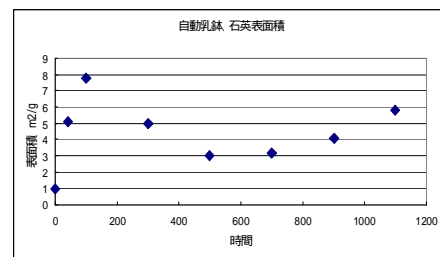
図2. 磨砕時間と表面積変化
