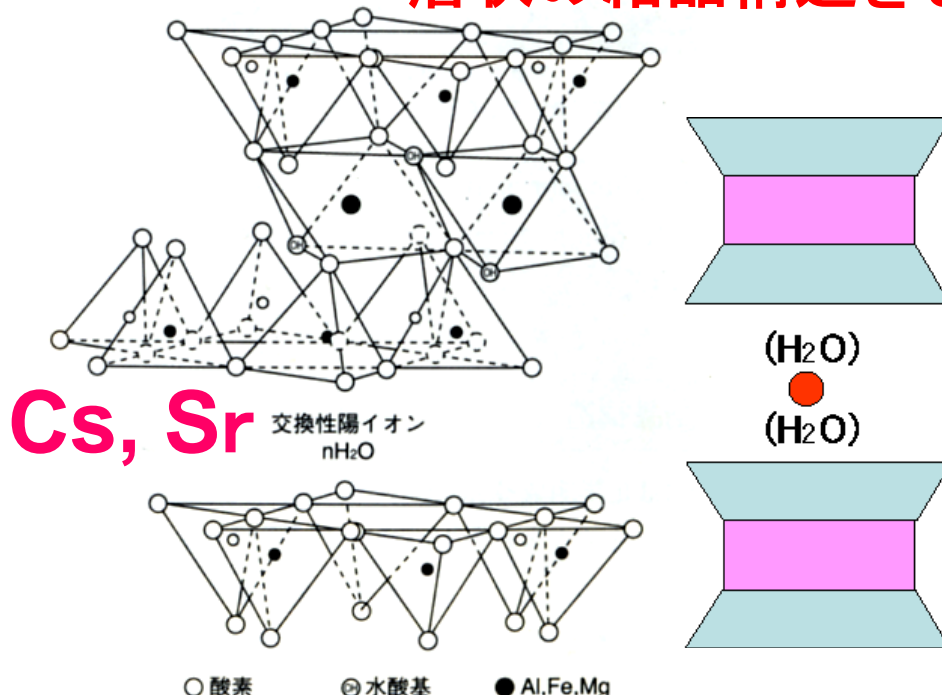
図2-1 モンモリロナイトの結晶構造 1)
