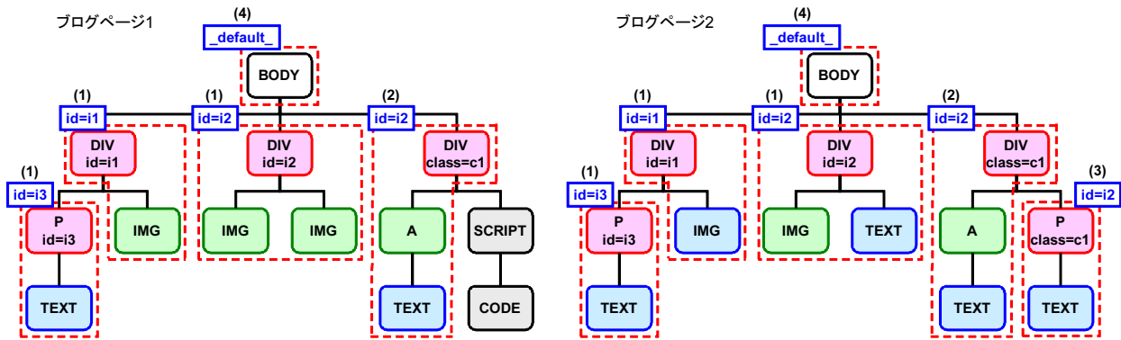
図2 DOM ツリー（要素識別子は要素内に記載）からのブロック抽出（破線枠部分、計 11 ブロック）及び各ブロックに位置ラベル（実線矩形枠部分）を付与した例．ブロック抽出の際は、SCRIPT、NOSCRIPT、STYLE の 3 要素をブロックに含めない他、BODY 要素は例外的にブロックとして認める．位置ラベル上部の括弧付き数字は、2.3 節に記載した位置ラベル付与規則を表す．たとえば、ブログページ 1 の「class=c1」は、両方のブログページ 1 において 2 度出現しているが、ブログページ 2 において 2 度出現しているため、規則 (1) は適用されず、規則 (2) が適用される．
