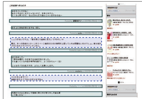
図3 従来手法には連続するコンテンツの一部を取りこぼすという欠点が存在する（破線矩形部分）．提案手法ではコンテンツブロック（実線矩形部分）の情報を用いて、コンテンツとして取りこぼしたブロックを再抽出する．
