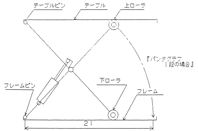
図 3 2 2 実行結果 (パンタグラフ1段)
