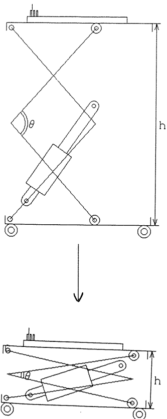
図 3 2 1 実行結果 (テーブルリフタ)
