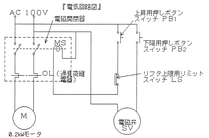
図 3 2 3 実行結果 (電気回路図)
