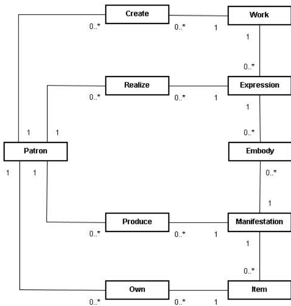
図1 プロトタイプシステムでの要素と関連
