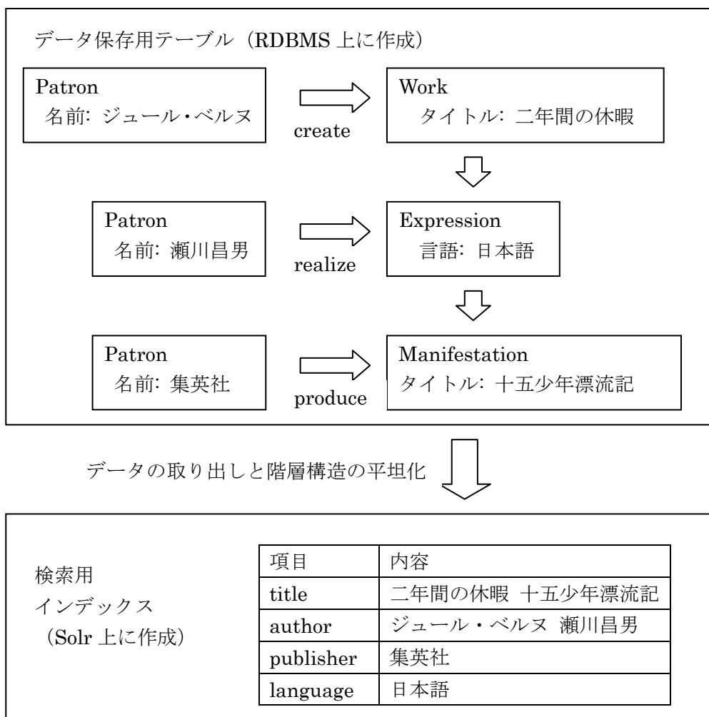
図2 RDBMS と Solr でのデータの保持
