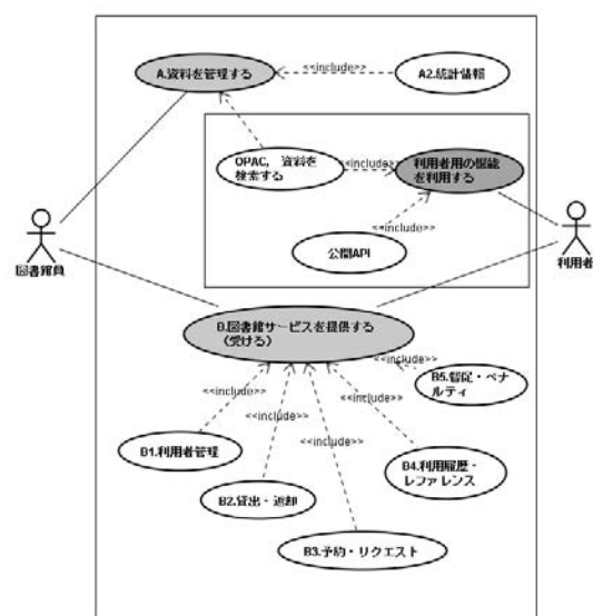
図 9. UML で記述した仕様の例
