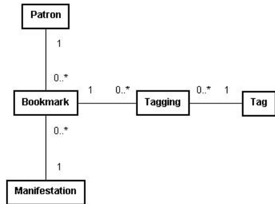
図7 ブックマーク・タグ・資料の関連
