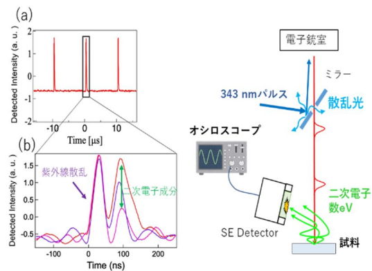
図2 検出される2次電子信号波形
