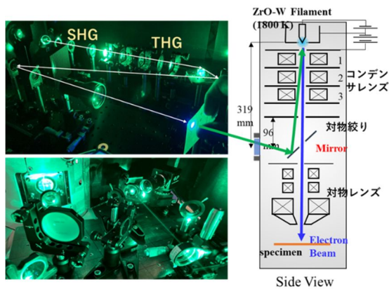
図1 フェムト秒レーザー光学系
