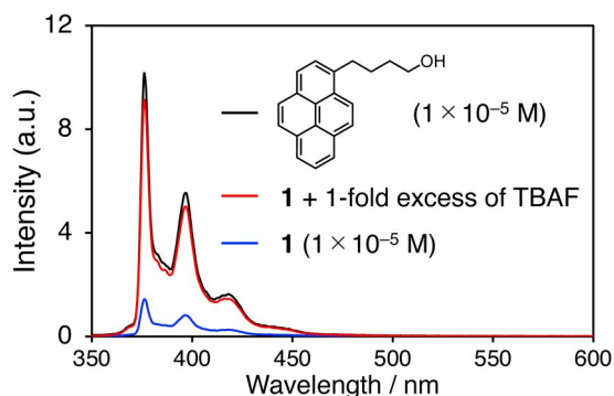
図 蛍光スペクトル：[2]-ロタキサンに対するフッ素アニオンの添加実験（溶媒：DMSO、 \lambda_{ex}=318 nm）
