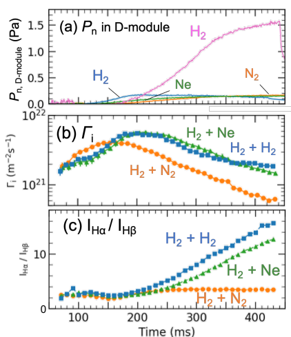
図 5: 水素ガスと少量の窒素, ネオン, 水素の重畳入射時の(a)中性ガス圧, (b)ターゲット板静電プローブ #3 におけるイオン粒子束, (c) H\alpha 線と H\beta 線強度比。
