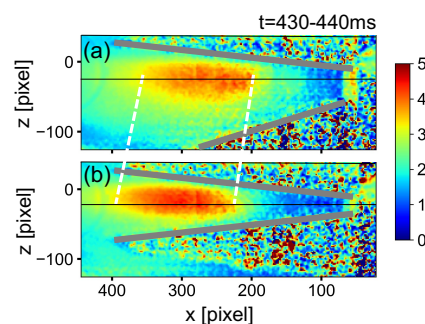
図 7: H_2 入射時の V 字ターゲット角度の違いによる H\alpha, H\beta 線発光強度比空間分布の比較。ターゲット開口角 (a) 約 40 度, (b) 約 15 度。
