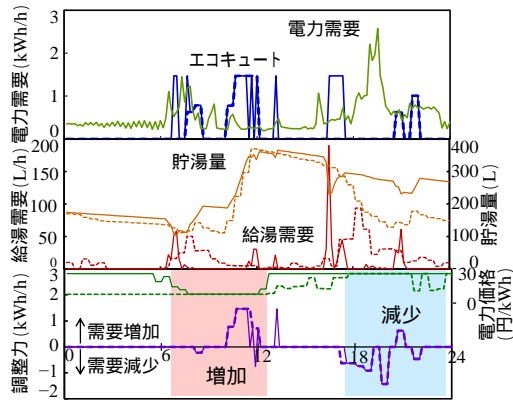
図4 CO2HP の運用
