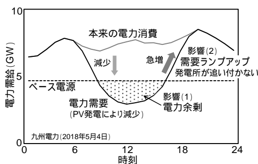
図 1 PV 普及による電力系統への影響
