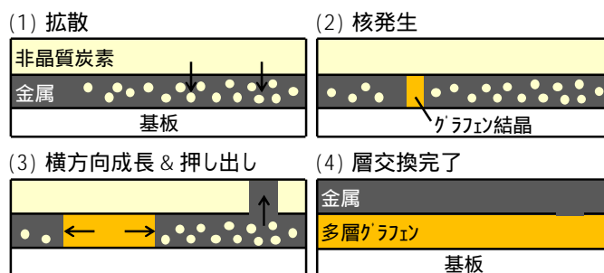
図1. 層交換現象のメカニズム概要
