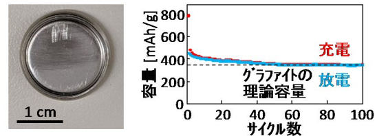
図 4. 作製したコイン電池とサイクル特性
