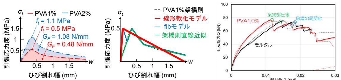
図8 FEAにおけるDFRCCの引張モデル
