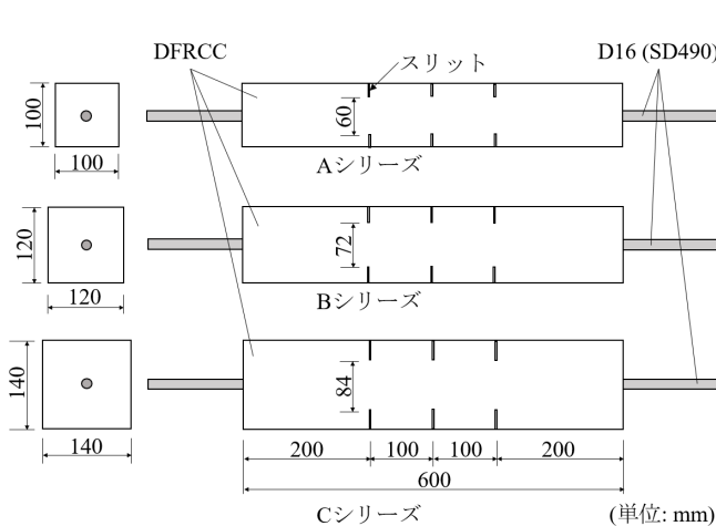
図4 鉄筋併用 DFRCC 要素の一軸引張試験試験体
