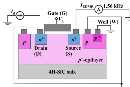
図1 SiC-MOSFET と、EDMR 分光セットアップ (文献[1]より一部変更して転載)。
