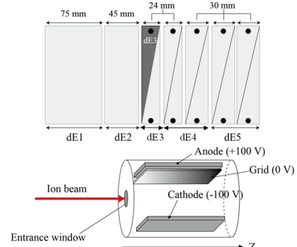
図 2 5 枚電極型ガス \Delta E-E 検出器の構成
