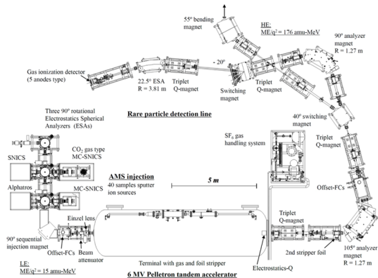
図 1 6 MV 加速器質量分析装置の概略図
