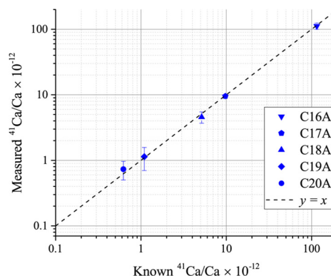
図4 ^{41}\text{Ca} -AMSの検量線
