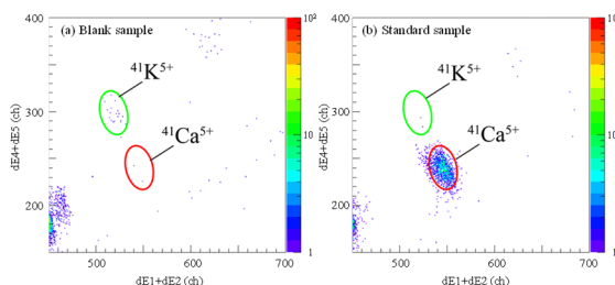
図3 ^{41}\text{Ca} の2次元スペクトル図 (a) ブランク試料、(b) 標準試料 ^{41}\text{Ca}/^{40}\text{Ca} = 1.16 \times 10^{-10}
