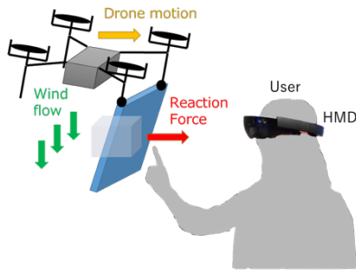
図 5 : 柔軟シートによる水平方向への力覚提示
