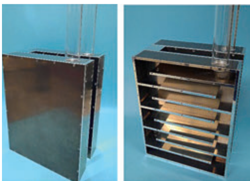
呼気冷却装置 (右：内部の冷却構造)
