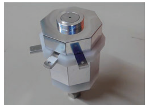
吸収電流測定用積分球
