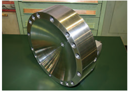
水中音響反射鏡
