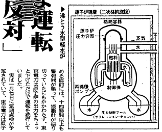
原子炉構造(二次冷却炉型)
