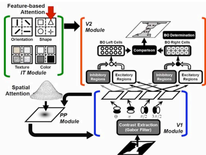
図 1. 図方向細胞の群化が、空間的注意と特徴に基づく注意によって変調され、知覚される図・形状が変化するモデル。
